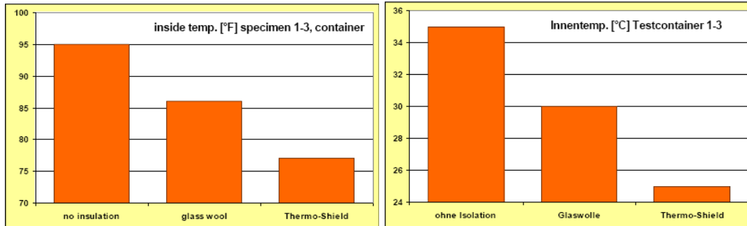
Bild 02: Lägre inomhustemperatur i den termoskydd-behandlade containern jämfört med både den isolerade och den oisolerade containern [°C].
