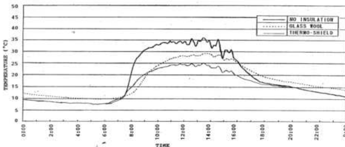
Bild 01: Temperaturkurvor under hela testet visade maxtemperaturen Uppifrån och ner ingen isolering (~35°C), mineralull (<30°C), Termoskydd (<25°C)
